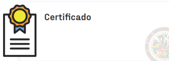
Figura 11. Generar Certificado
